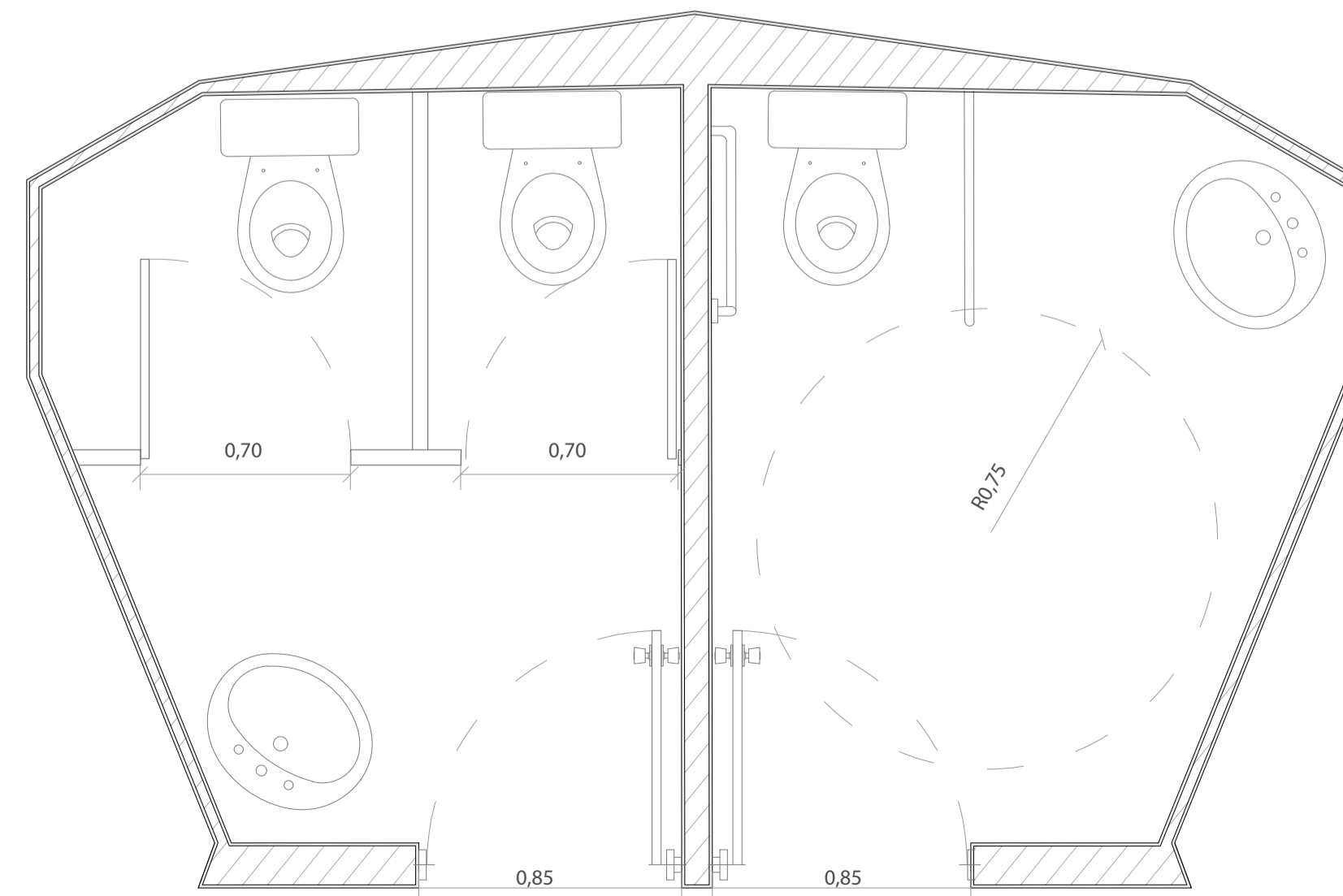
MÓDULO DE BAÑO PREFABRICADO área: 10m 2
